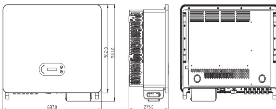
Figura 4 - Vista anteriore, laterale e posteriore dell'inverter (3PH 80KTL-V3)
