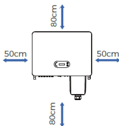
Figura 14 - Spazio libero per un singolo inverter
