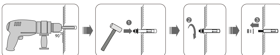
Figura 19 - Inserimento delle viti nei fori
