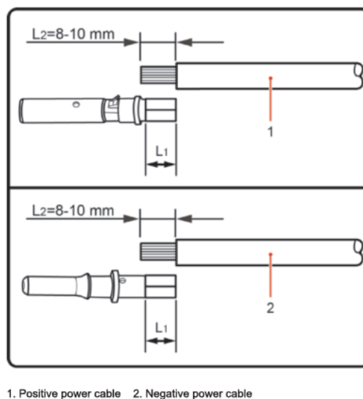
Figura 28 – Collegamento dei cavi di alimentazione in ingresso CC (1)
